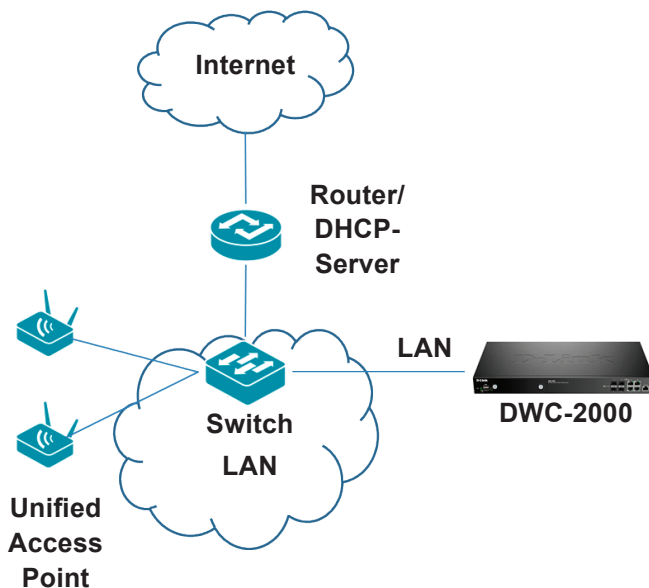
Abbildung 10. Netzwerktopologie
